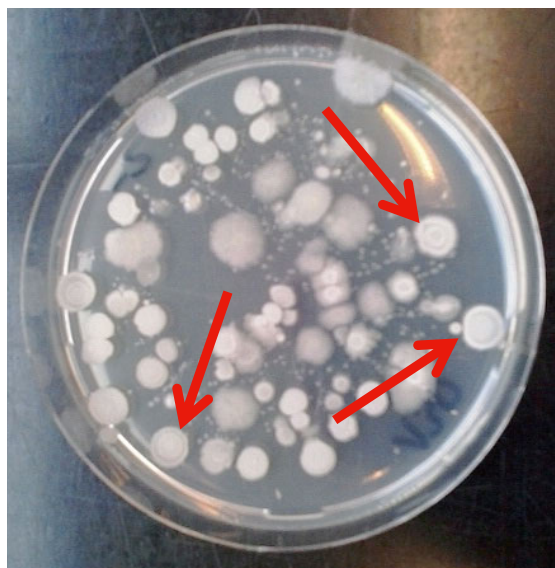
Abbildung 2: Plate-Count-Agarplatte mit Bacillus spp. Kolonien (rote Pfeile).
